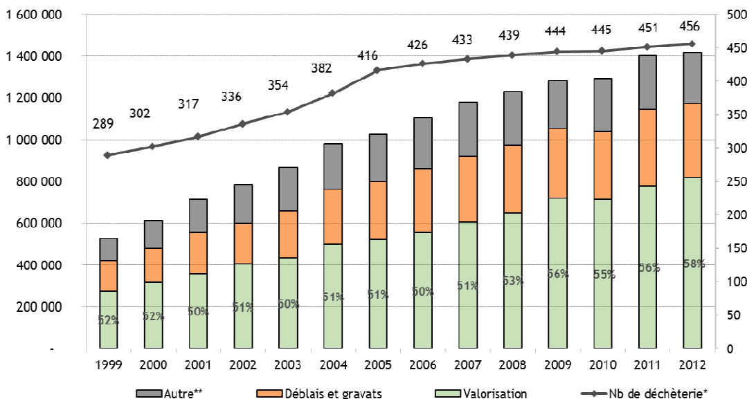
Evolution du nombre de déchèteries et des tonnages reçus de 1999 à 2012
